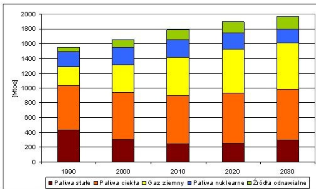
Rys. 2. Zapotrzebowanie Unii Europejskiej na energię do 2030 r.
